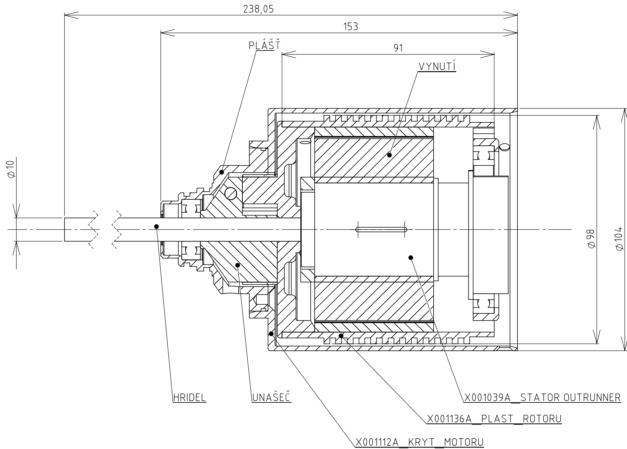
ŘEZ A-A
